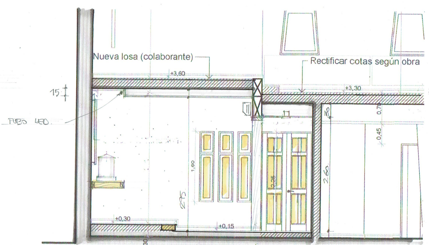
TERMINACIONES INTERIORES ESC 1:50
